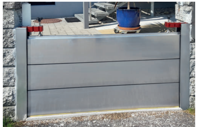
Hochwasserschutzzaun
