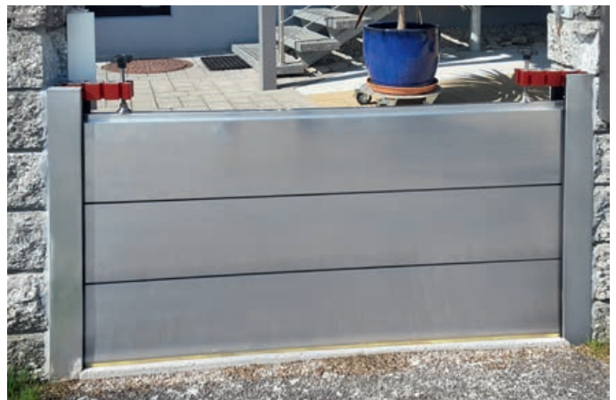
Hochwasserschutzzaun
