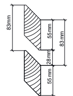
45° abgeschrägt/ 45° biseauté
