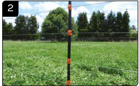
2 Bestimmen Sie die richtige Drahthöhe
